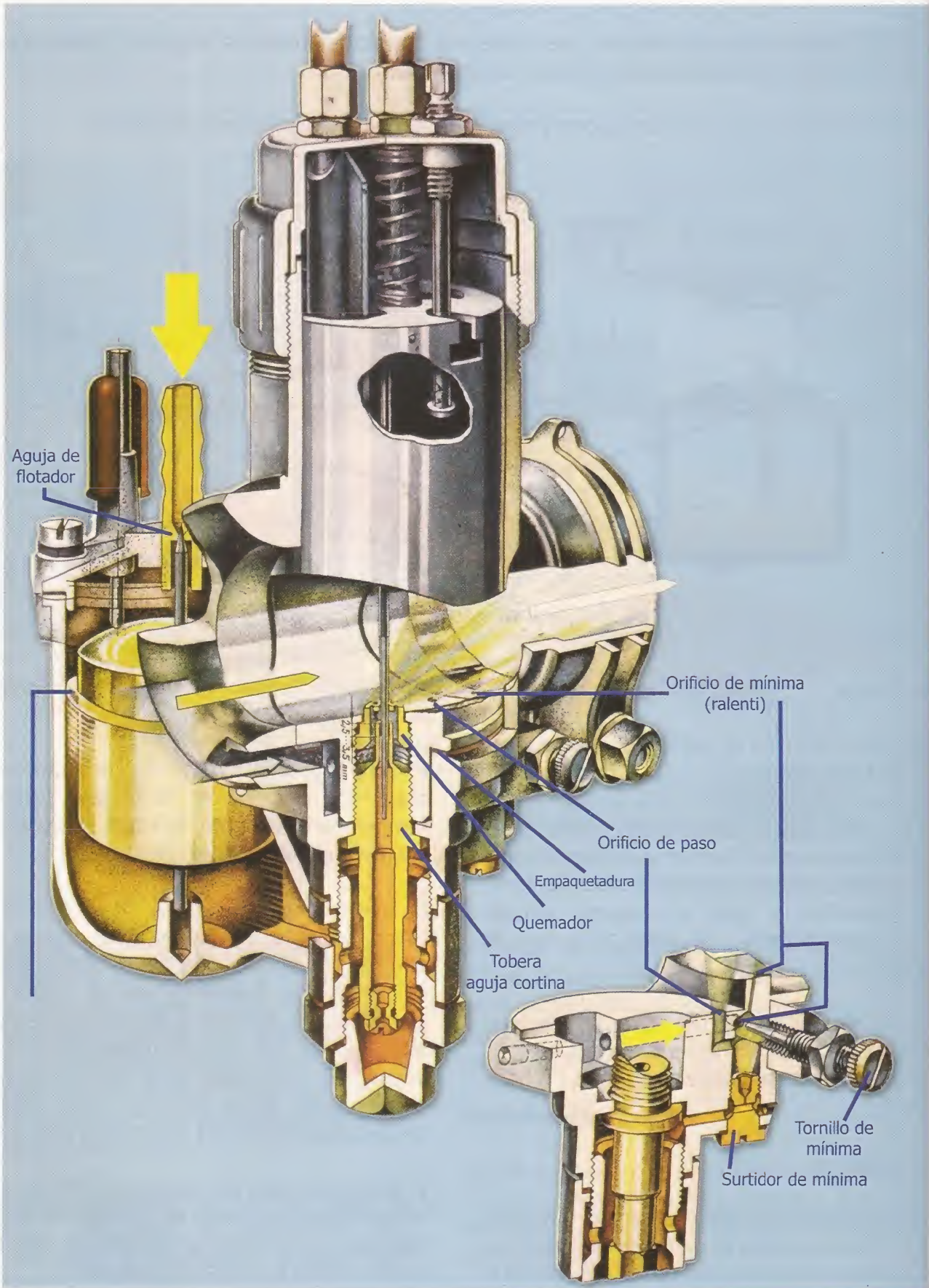
Corte de carburador tipo KNB
